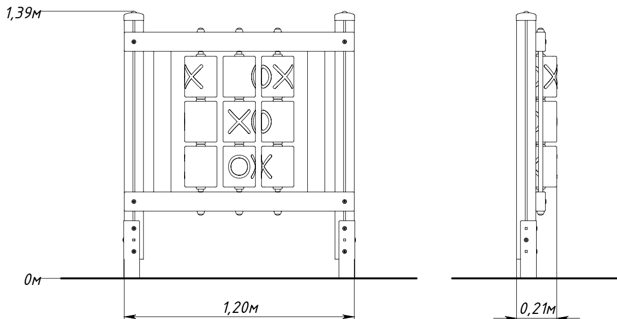
Рисунок 1 — Основные габаритные размеры
