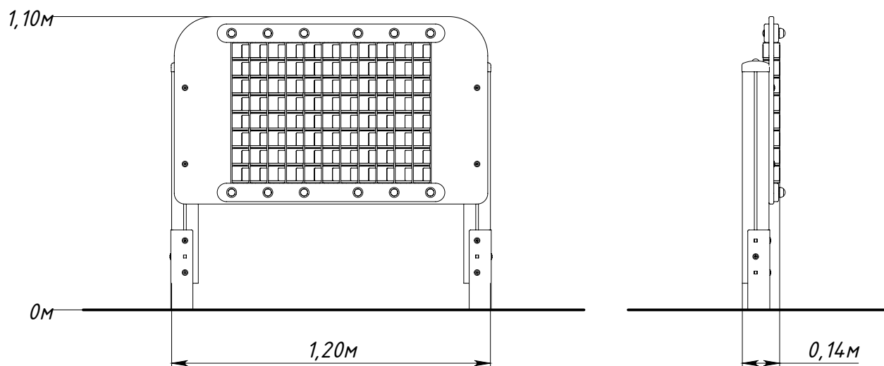
Рисунок 1 — Основные габаритные размеры
