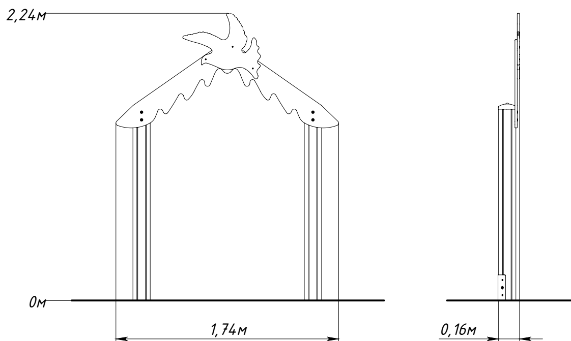
Рисунок 1 — Основные габаритные размеры
