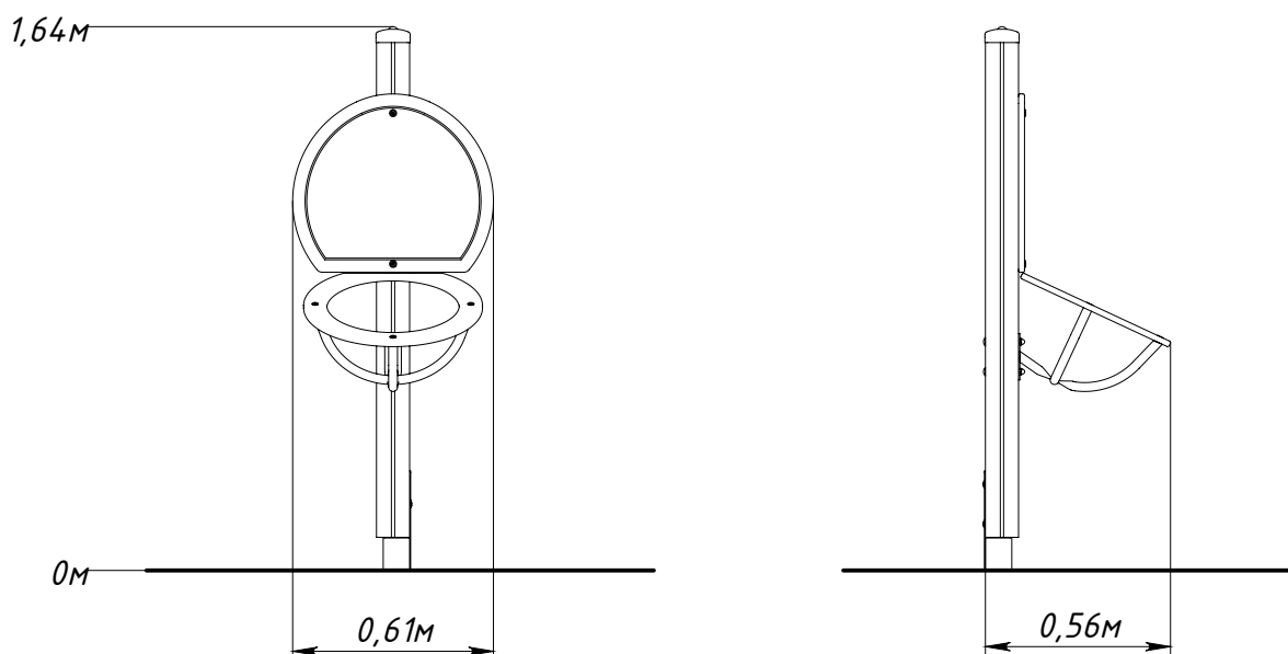
Рисунок 1 — Основные габаритные размеры
