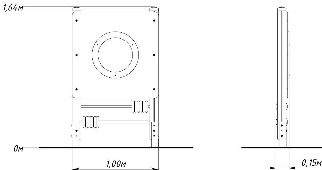
Рисунок 1 — Основные габаритные размеры
