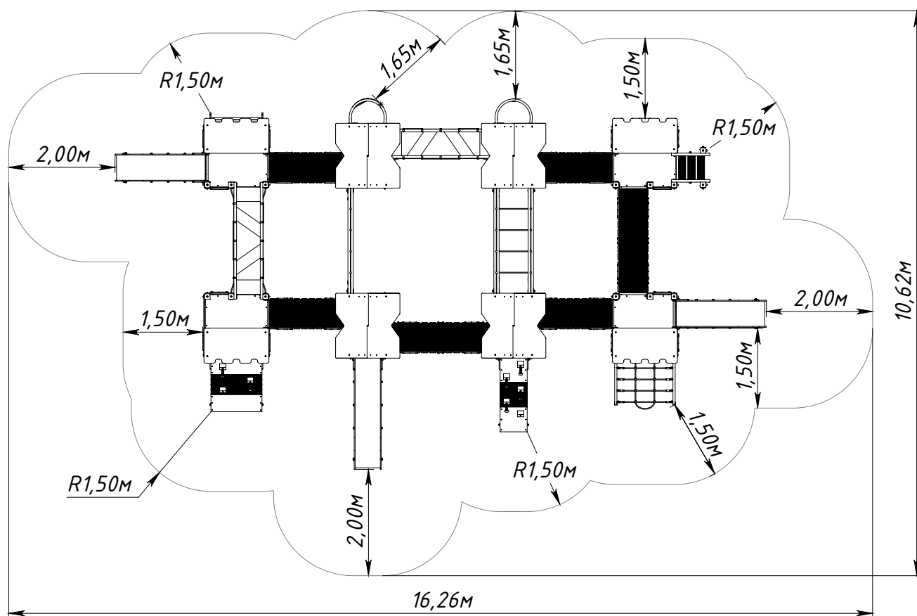
Рисунок 2 — Граница зоны приземления
