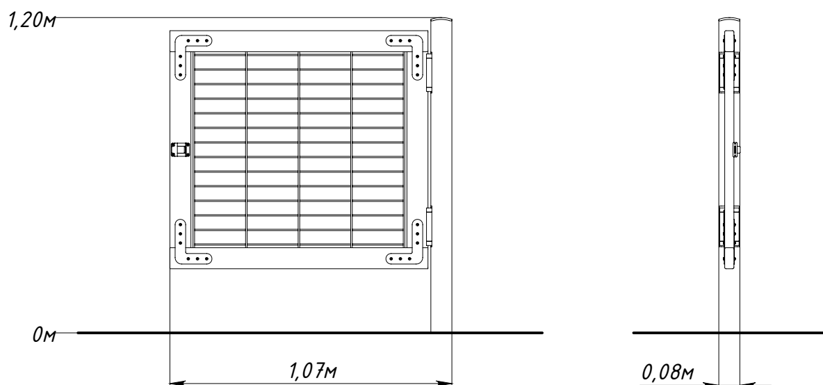
Рисунок 1 — Основные габаритные размеры
