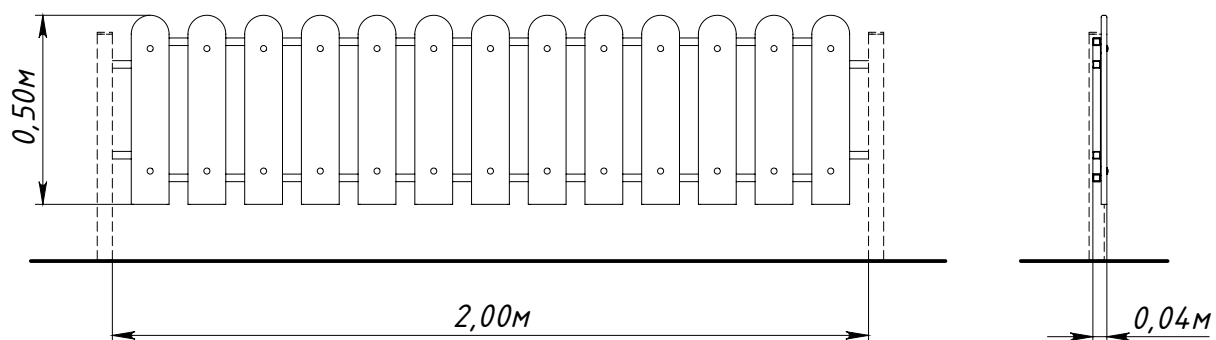
Рисунок 1 — Основные габаритные размеры
