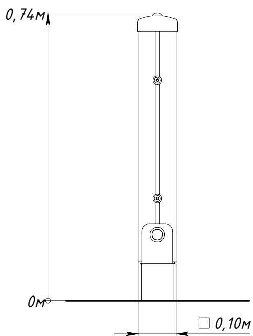
Рисунок 1 — Основные габаритные размеры
