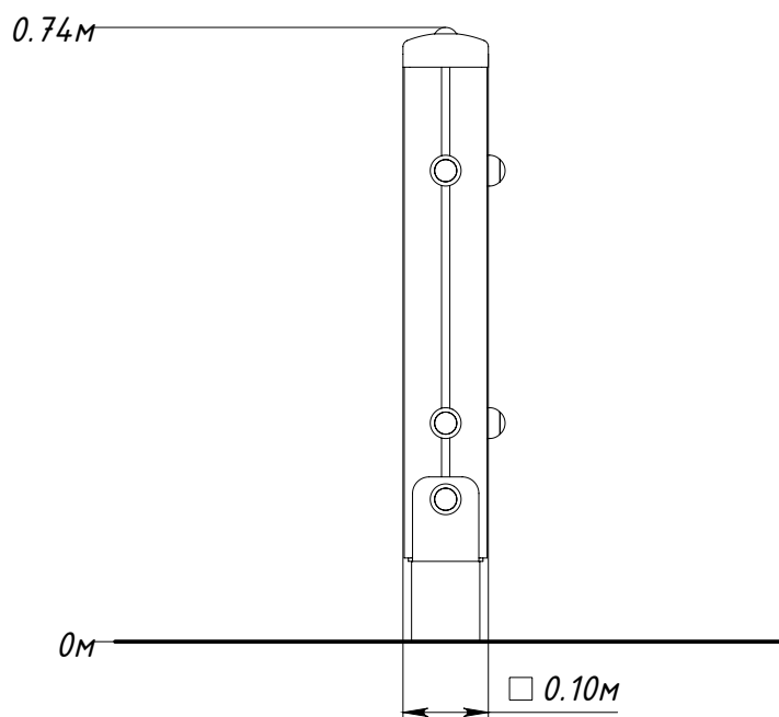
Рисунок 1 — Основные габаритные размеры
