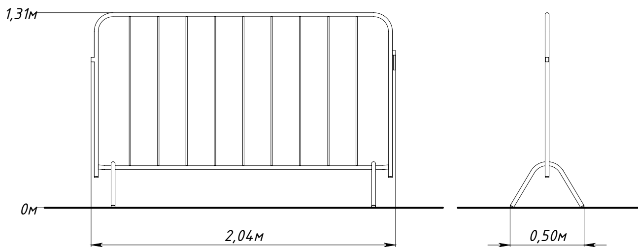
Рисунок 1 — Основные габаритные размеры
