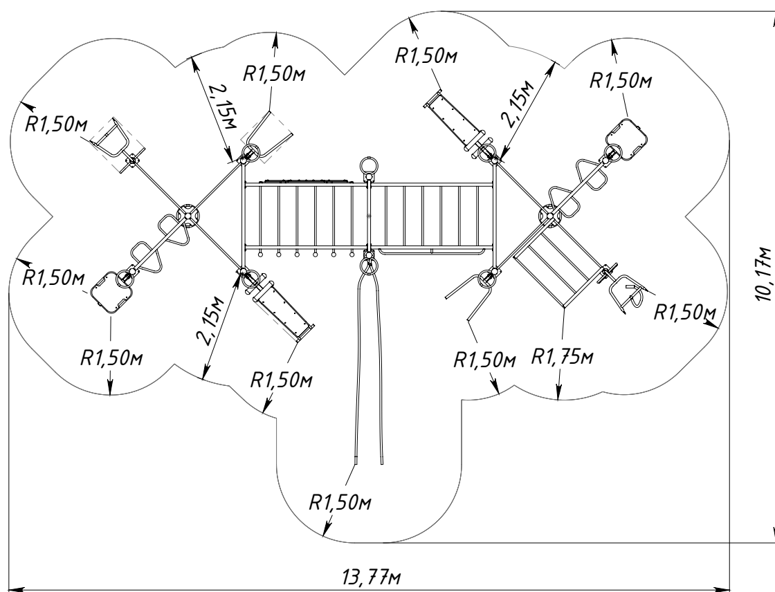
Рисунок 1 — Основные габаритные размеры
