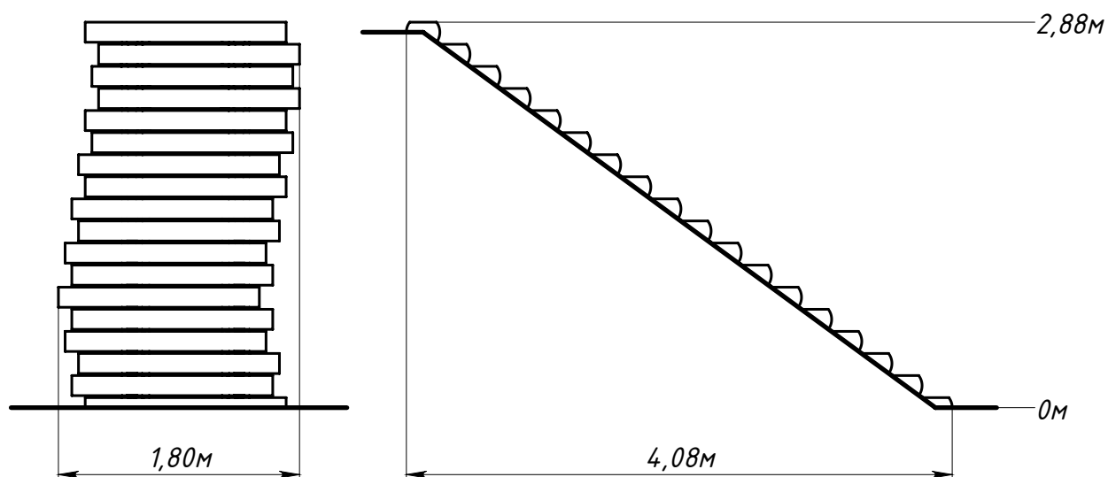
Рисунок 1 — Основные габаритные размеры
