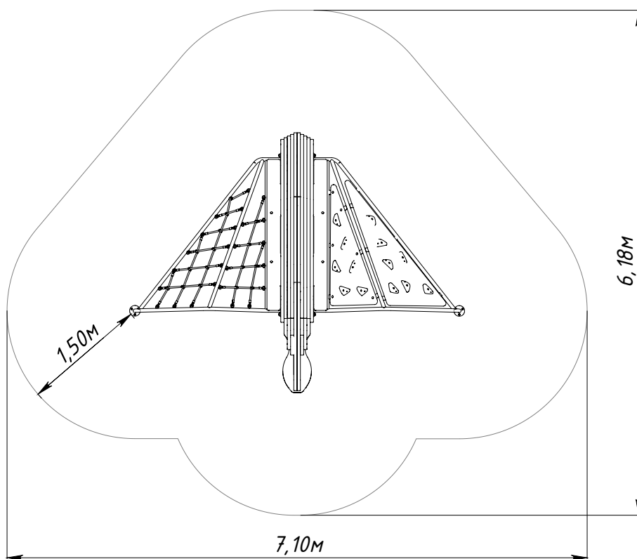
Рисунок 1 — Основные габаритные размеры
