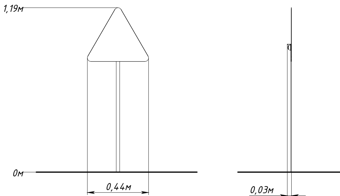
Рисунок 1 — Основные габаритные размеры
