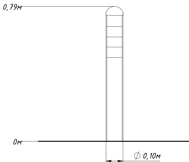
Рисунок 1 — Основные габаритные размеры
